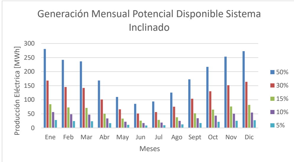
Figura 28. Generación Mensual Sistema Inclinado Según Impacto.
