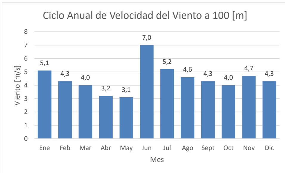
Figura 9. Velocidad del Viento [15].
