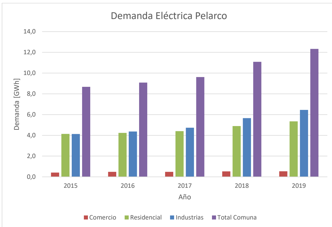
Figura 17. Demanda Eléctrica Pelarco [17].
