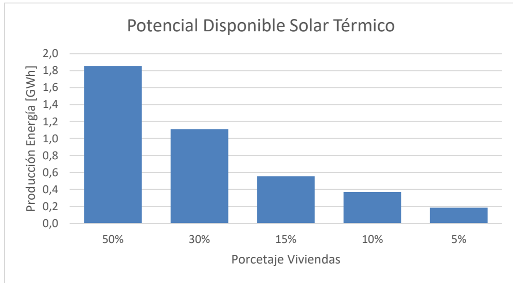
Figura 29. Potencial Disponible Térmico Solar Según Impacto.
