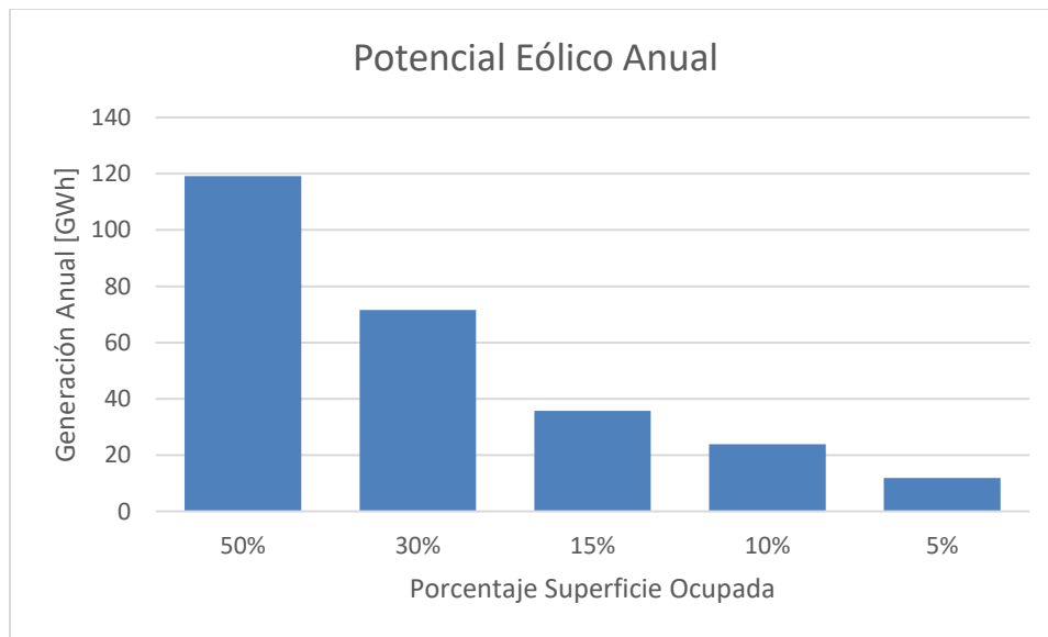
Figura 31. Generación Eólica Según Superficie Ocupada.
