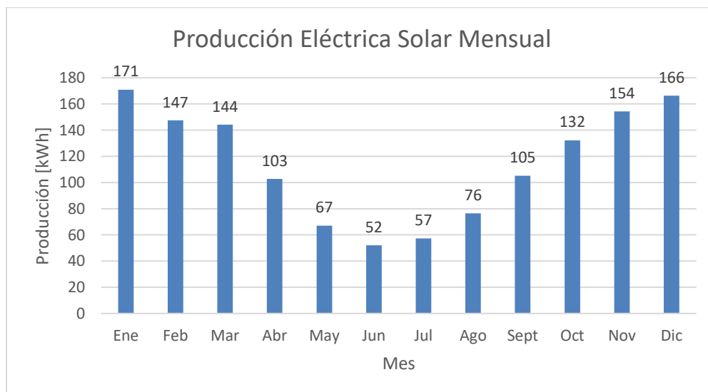
Figura 26. Producción Energética Mensual [37].
