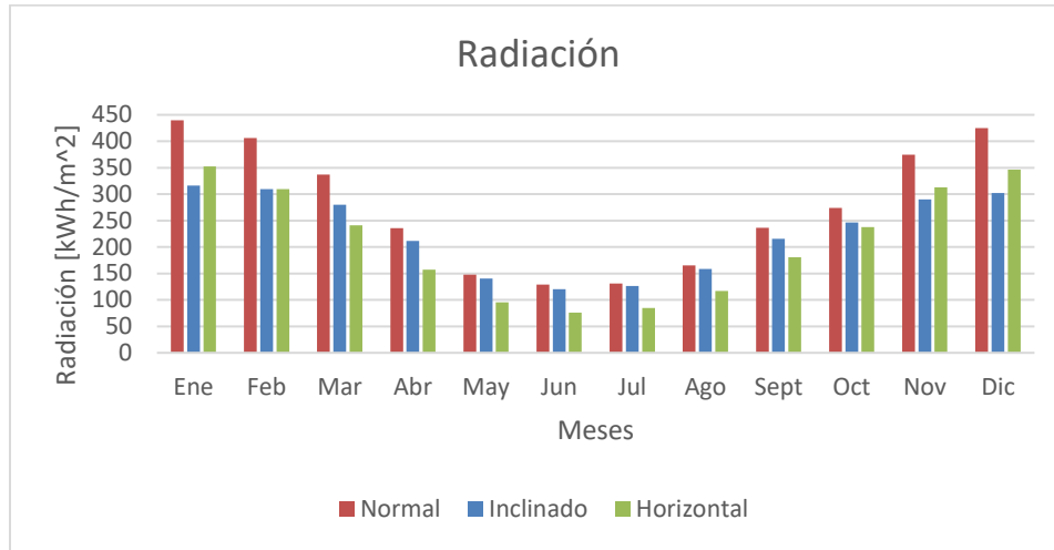
Figura 25. Radiación Diferentes Disposiciones [37].
