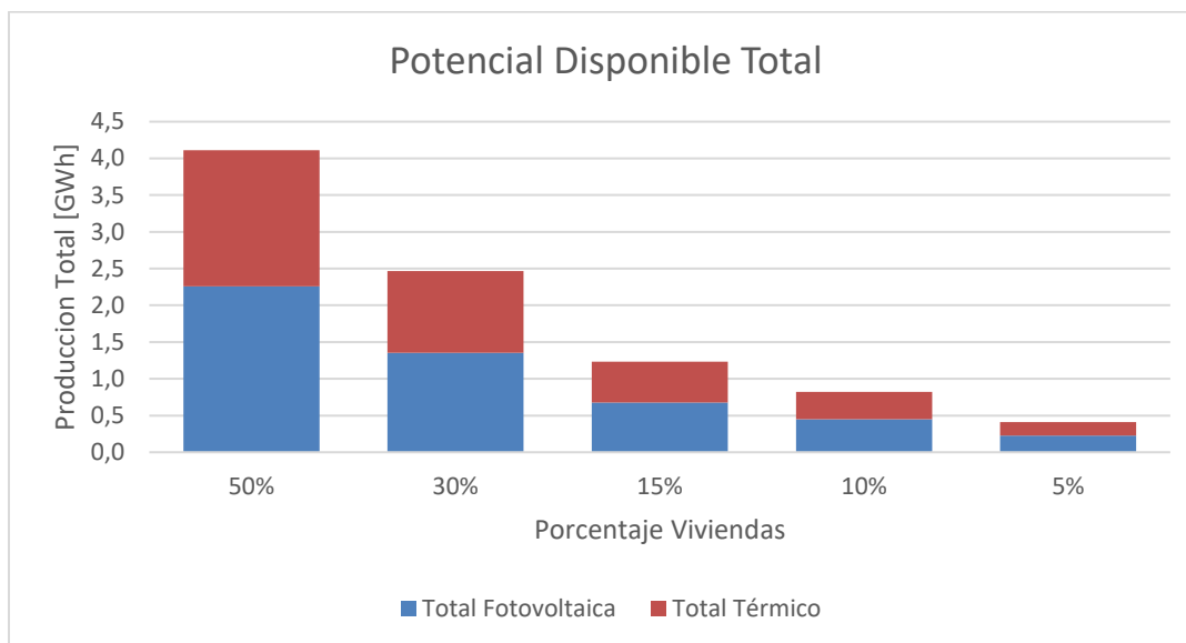
Figura 30. Potencial Disponible Total Solar Según Impacto.
