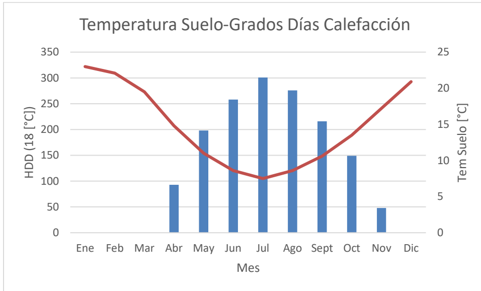
Figura 8. Temperatura Suelo-Grados Días Calefacción [14].
