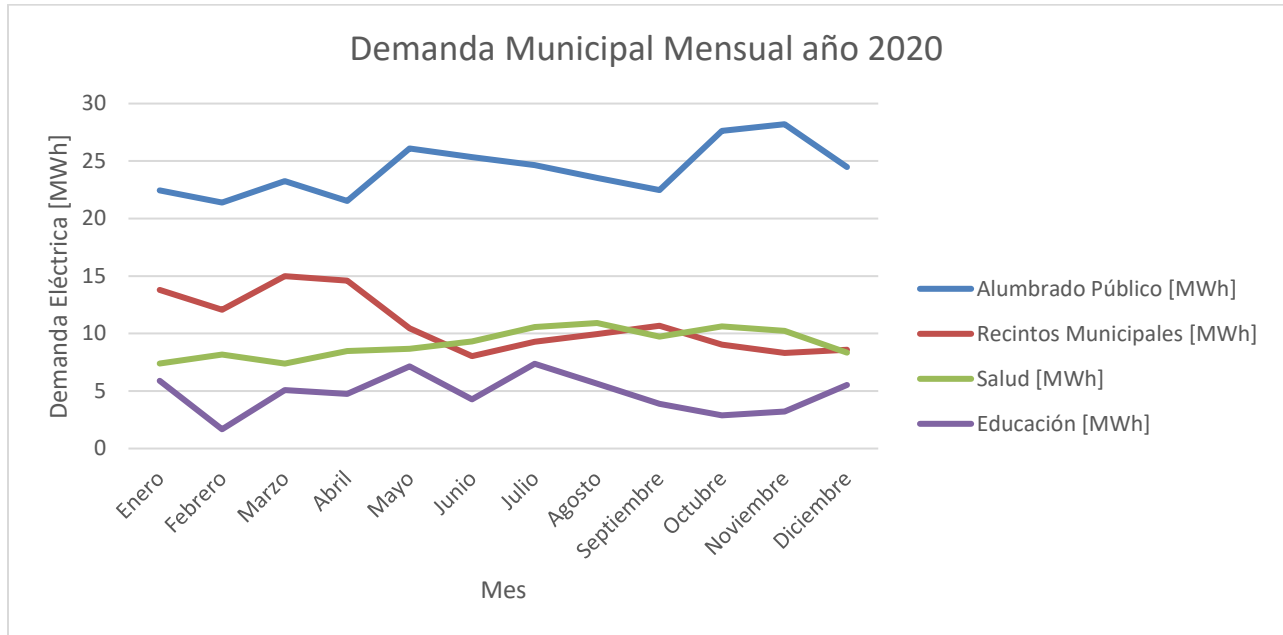
Figura 19. Demanda Eléctrica Municipal Mensual.
