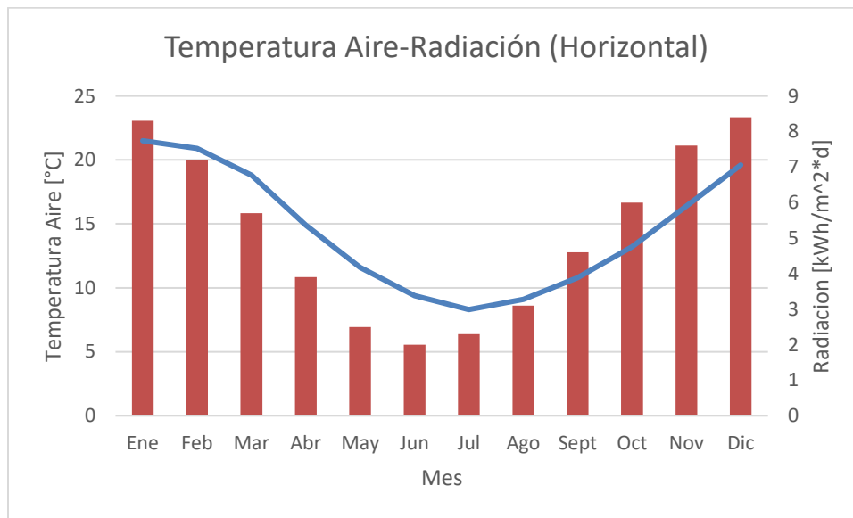
Figura 7. Temperatura Aire-Radiación (Horizontal) [14].
