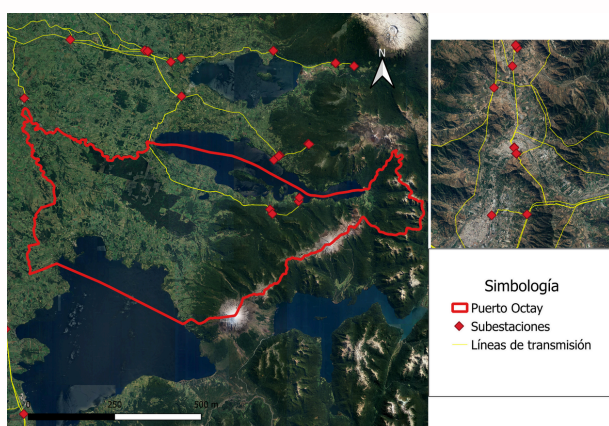
Figura 12. Ubicación de subestación eléctrica y líneas de transmisión en la comuna de Puerto Octay.
