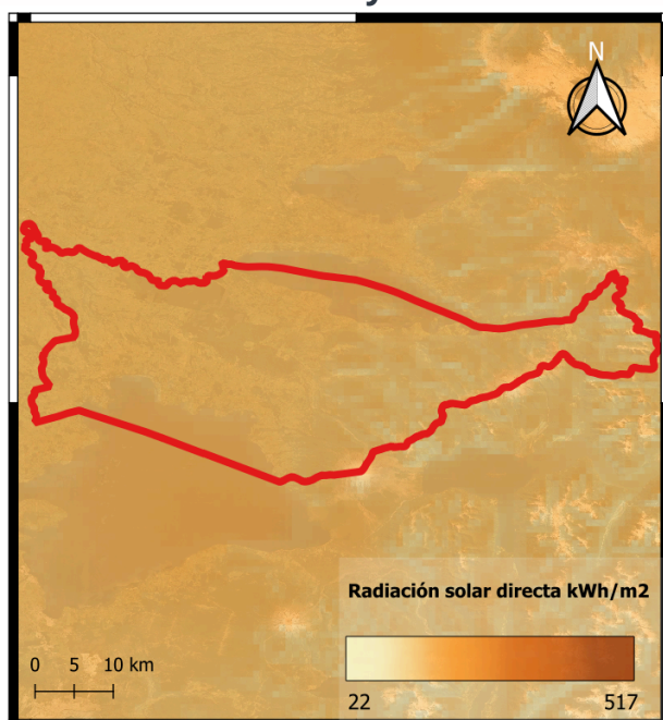
Figura 24. Radiación solar en Puerto Octay.
