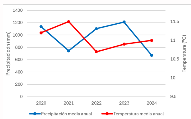
Figura 11. Precipitación y temperatura media anual de los últimos 8 años en la comuna de Puerto Octay.
