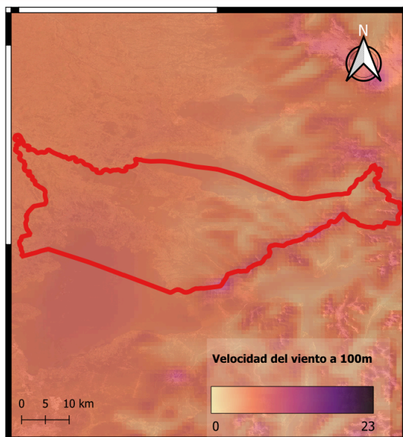
Figura 26. Velocidad del viento en Puerto Octay.
