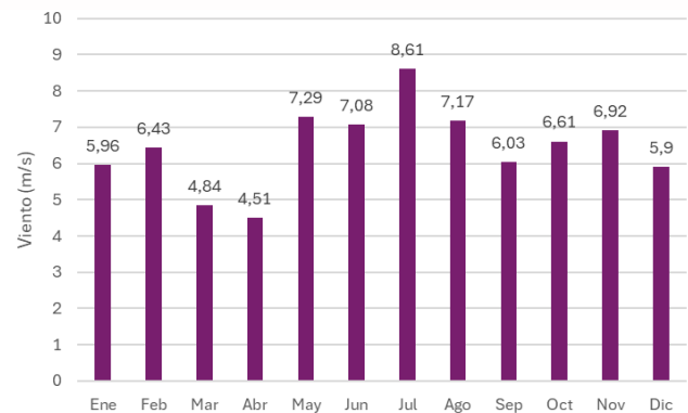
Figura 27. Velocidad del viento promedio mensual a 100 metros de altura en la comuna de Puerto Octay.
