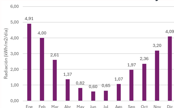
Figura 25. Promedios mensuales de Radiación Solar en Puerto Octay.
